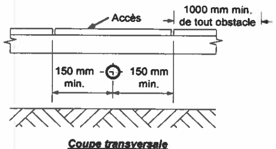
Montage dissimulé sous un plancher
