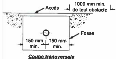
Montage dissimulé dans une dalle sur sol
