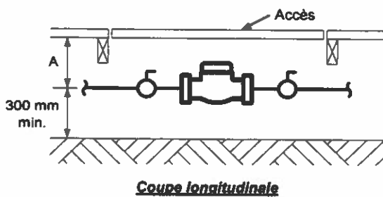
Montage dissimulé sous un plancher
