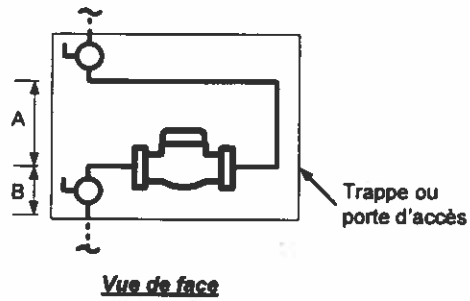
Montage dissimulé dans un mur
