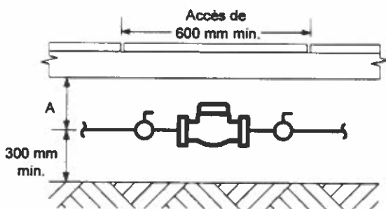
Montage en retrait dissimulé sous un plancher
