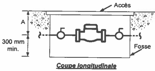
Montage dissimulé dans une dalle sur sol
