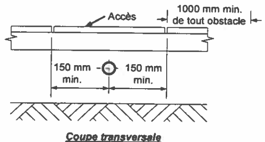
Montage dissimulé sous un plancher
