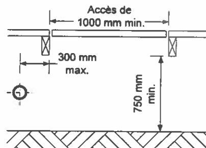
Montage en retrait dissimulé sous un plancher
