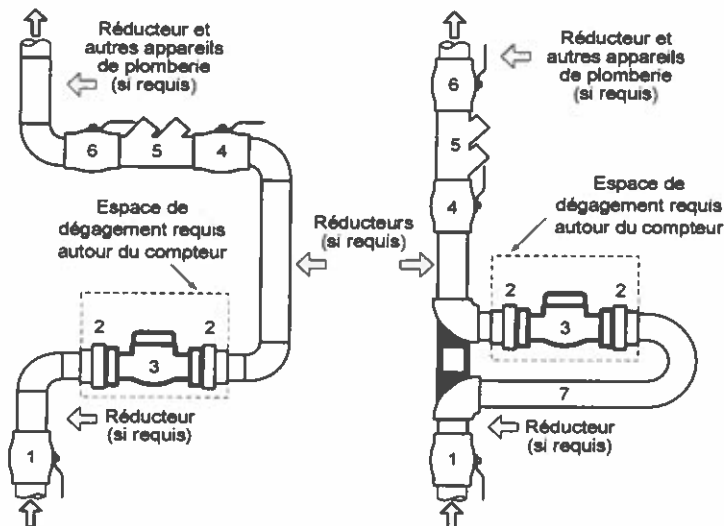
MONTAGE VERTICAL (Aucune échelle)
